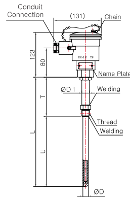
Model No. | SS-5013E (Metal Protection Tube)
