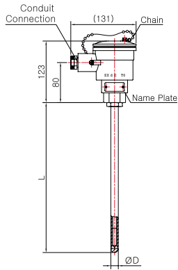
Model No. | SS-5011E (Metal Protection Tube)
